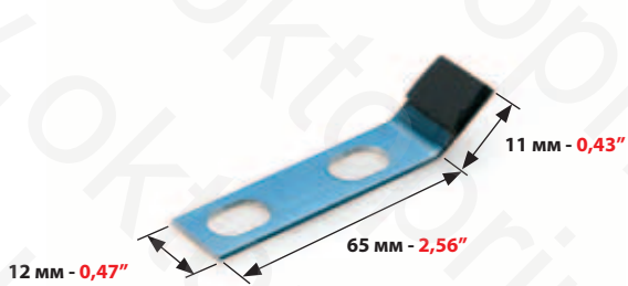
ВЫХОДНОЙ ГРЕЙФЕР ДЛЯ ТИГЕЛЬНЫХ МАШИН ДЛЯ: EXIT GRIPPER FOR LETTERPRESS MACHINE FOR: HEIDELBERG CYLINDER
