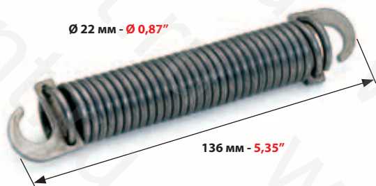
ПРУЖИНА ДЛЯ СТАЛКИВАТЕЛЯ ЛИСТА ДЛЯ: SPRING FOR FEED JOGGER LEVER FOR: HEIDELBERG GTO 46/52/SPEEDMASTER 102
