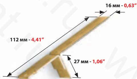
ТОРМОЗ ЛИСТА ДЛЯ: SHEET STOP GUIDE FOR: HEIDELBERG GTO 46/52
