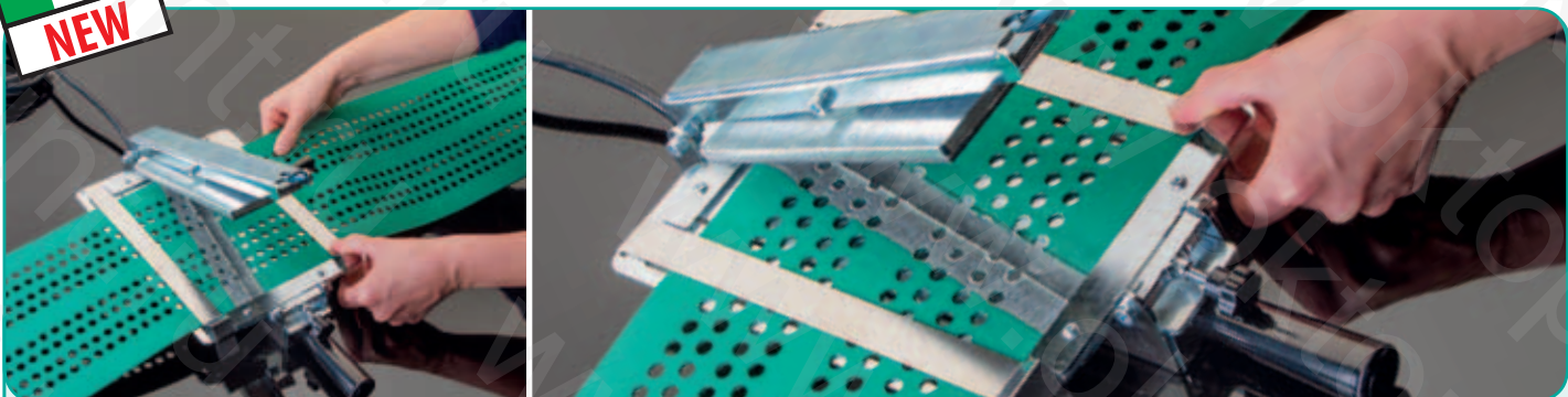
МАШИНКА ДЛЯ СКЛЕЙКИ ЛЕНТ ШИРИНОЙ ДО 200 MM WELDING MACHINE FOR FEEDER BELTS MAXIMUM WELDING WIDTH MM 200
